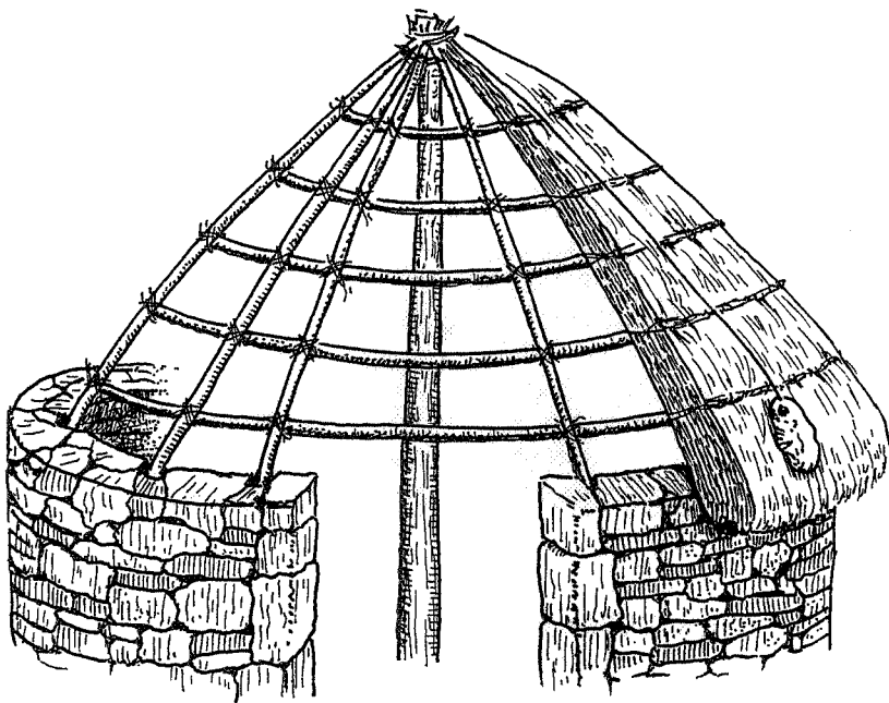
Detalle da construción do tellado
